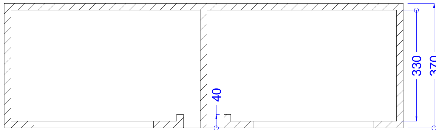
Seção A-A
